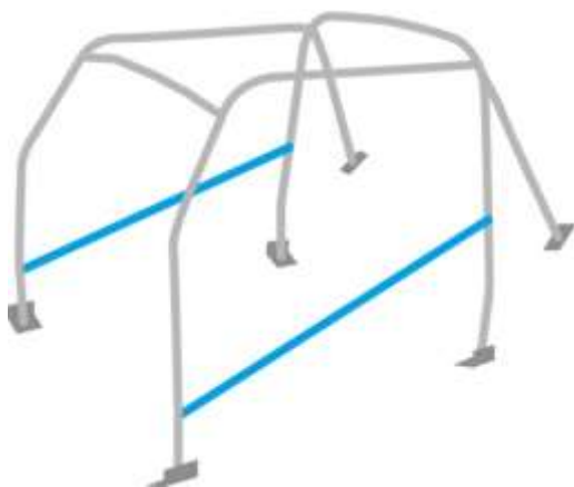
■6点式ロールケージと追加サイドバー(水色部)
